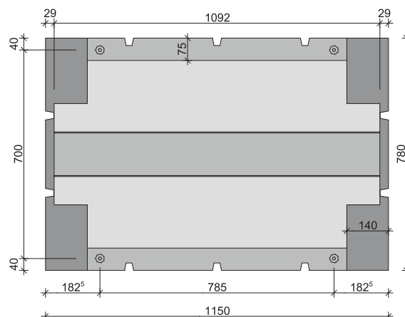
Ansicht Stirnseite
