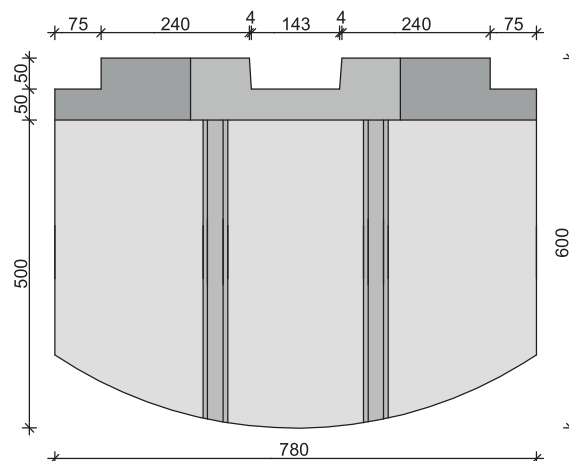
Ansicht Stirnseite
