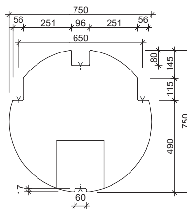
Ansicht Stirnseite
