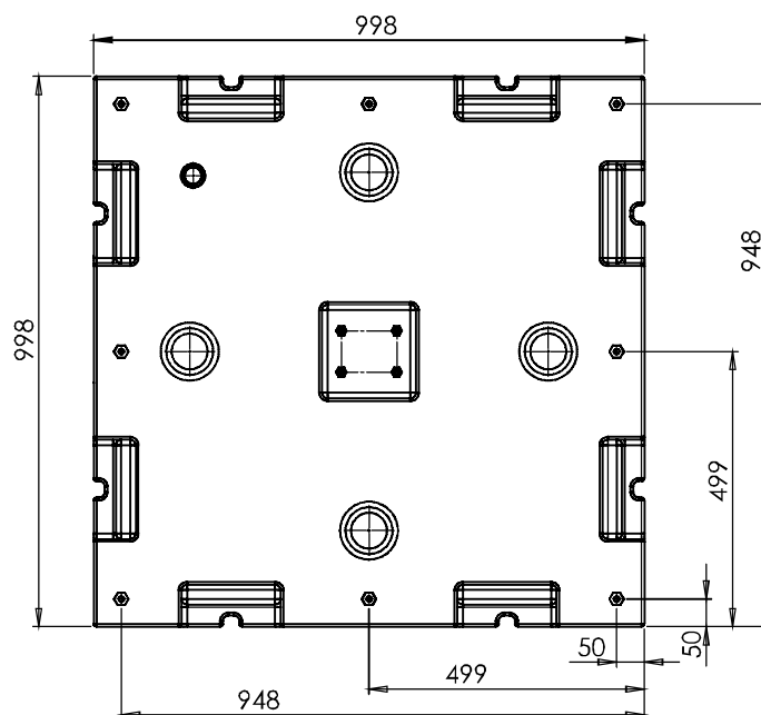
Draufsicht
